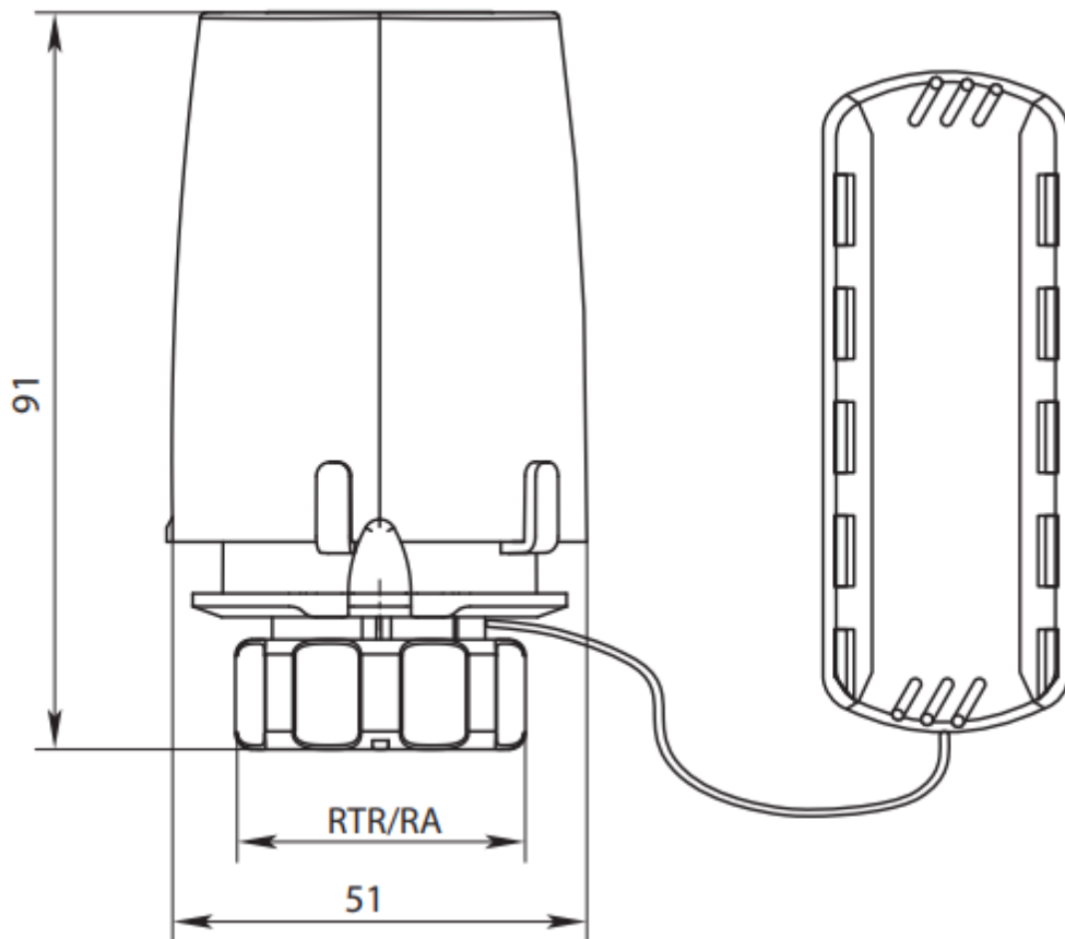
Рис. Габаритные размеры термoeлементa
